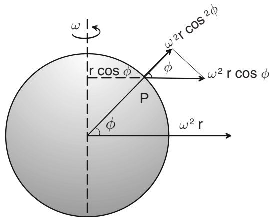
Figure 2.2 - Composantes de l’accélération centrifuge en un point P (latitude \phi ) sur la surface de la Terre (sphérique de rayon r ) en rotation avec une vitesse angulaire \omega .
