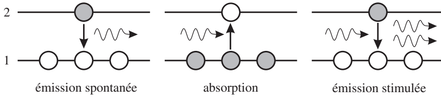
Figure 1.2 - Modèle d'Einstein. Les flèches ondulées désignent des photons. L'atome en grisé, après la transition, vient augmenter la population d'atomes « blancs ».
