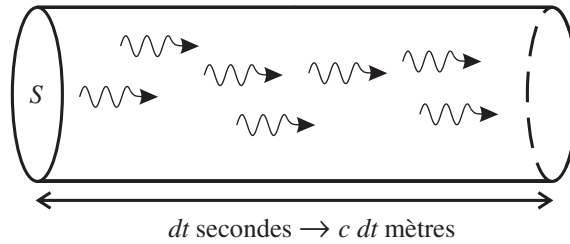
Figure 1.3 - Les photons, représentés ici par des flèches ondulées, se propagent dans une direction perpendiculaire à la surface S . Ceux qui traversent S à l'instant t parcourent pendant le temps dt la distance cdt . Les photons qui ont traversé S pendant le temps dt occupent donc un volume Scdt .
