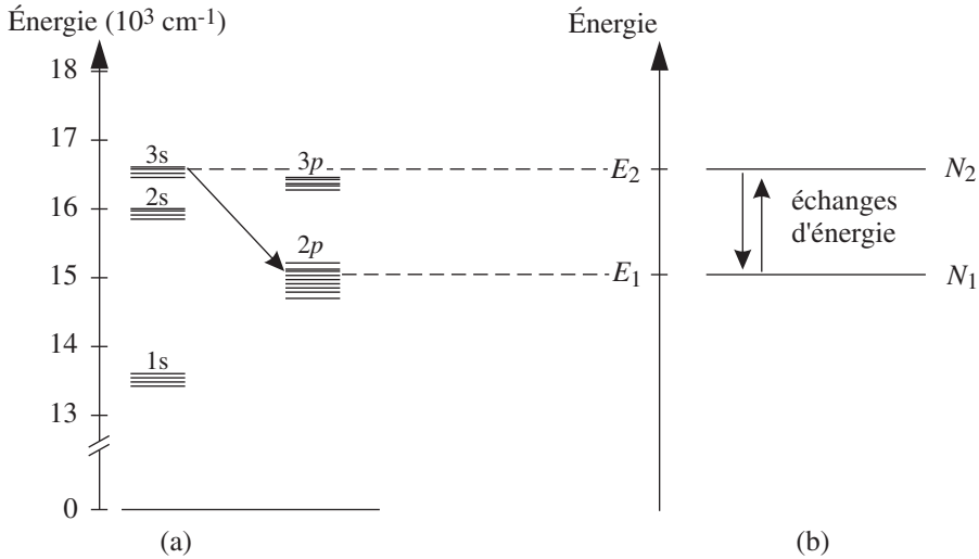
Figure 1.1 - Exemple de distribution d'énergie d'un atome ou d'une molécule. En (a), diagramme d'énergie de l'atome de Néon. Seuls quelques niveaux d'énergie électroniques sont représentés. La flèche indique la transition laser. En (b), diagramme d'énergie schématisé, ne retenant que les deux niveaux E_1 et E_2 de la transition laser.
