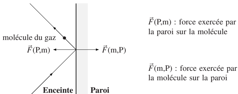
FIGURE 1.1 – Échange de quantité de mouvement entre une molécule de gaz et la paroi
