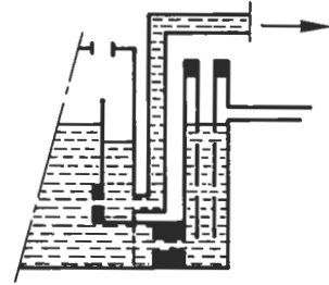
Fig. 19.4. Départ : débit supérieur à celui du gicleur.
