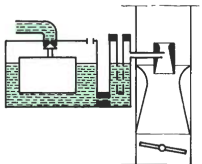
Fig. 16.15. La double buse favorise l'amorçage du circuit principal.
