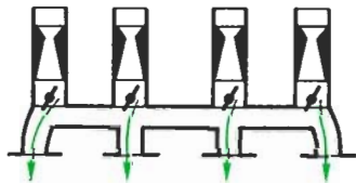
Fig. 18.8. Montage à deux carburateurs double corps.
