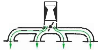
Fig. 18.6. Carburateur simple corps.
