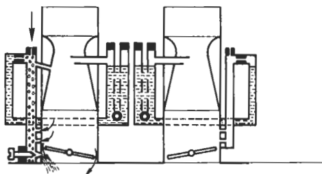
a) Ralenti.
