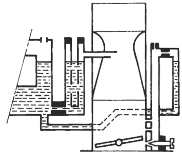
Fig. 17.6. Carburateur bijet.
