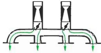
Fig. 18.7. Carburateur double corps à ouverture simultanée.
