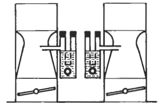
Fig. 18.5. Principe du carburateur à double corps.
