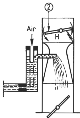
Fig. 19.2. ② Volet de départ.
