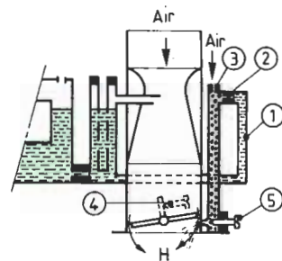
Fig. 17.2. Fonctionnement du ralenti.
