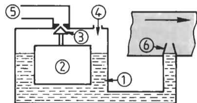
Fig. 16.2. Principe du niveau constant.
