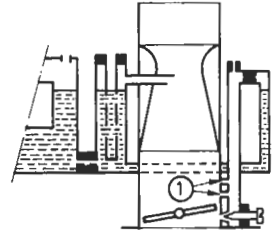
Fig. 17.3. Trous de progression (1).
