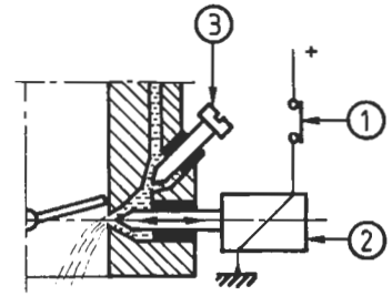
Fig. 20. 8. Electrovanne (étouffoir) de ralenti.
