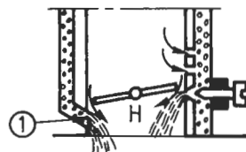
Fig. 19.1. ① Embouchure du circuit de starter.
