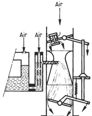
Fig. 19.8. Synchronisation du volet de départ et du papillon des gaz.
