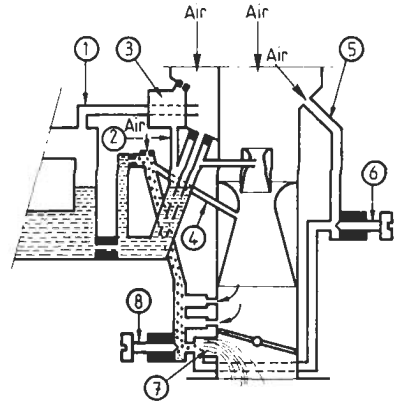
Fig. 20.4. Ralenti à balayage (Solex).
