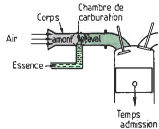
Fig. 16.1. Circulation de l'air et de l'essence.
