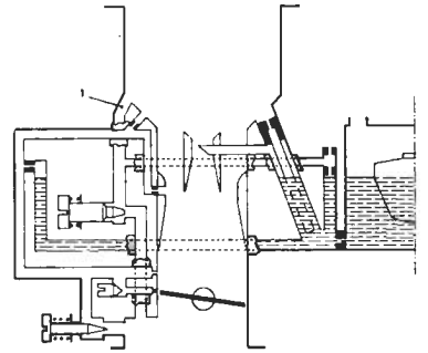
Fig. 20.5. Ralenti à richesse constante (document Solex).
