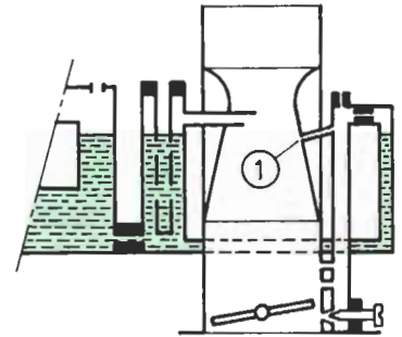
Fig. 17.5. Trou de non-renversement (1).
