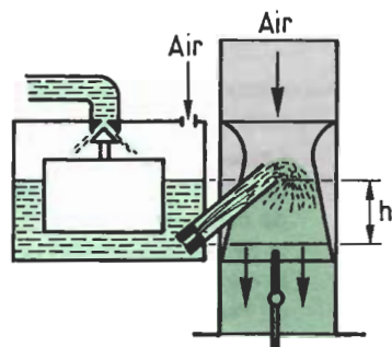
Fig. 16.9. Gicleur noyé. Capacité déjaugée.
