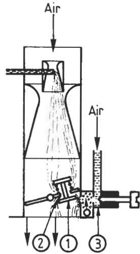
Fig. 20.6. Principe du décelateur (décel).
