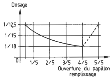
Fig. 16.7.b : Rappel de la courbe de dosage idéal.
