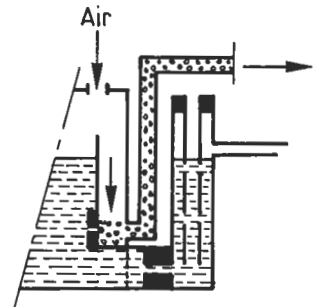
Fig. 19.5. Capacité déjaugée mise en dérivation du gicleur de starter.
