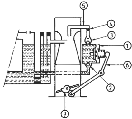
Fig. 18.1. Circuit de pompe de reprise.
