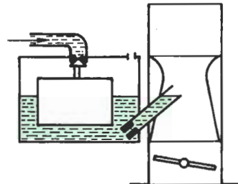
Fig. 16.8. Gicleur noyé.
