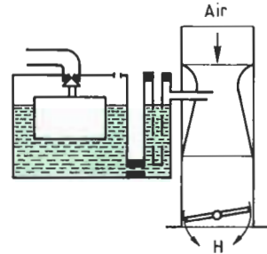
Fig. 17.1. Faible dépression. Amorçage du circuit principal impossible.
