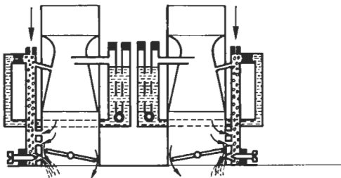
a) Ralenti.
