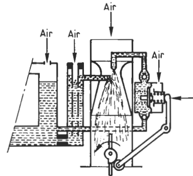
Fig. 18.2. Reprise.
