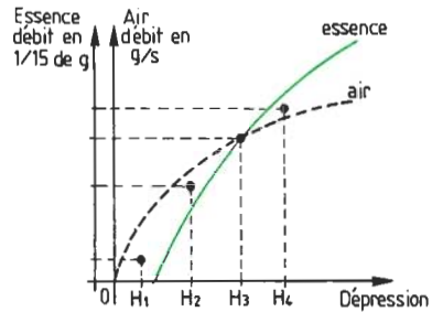
Fig. 16.7.a : Débit de l'air et de l'essence en fonction de la dépression.
