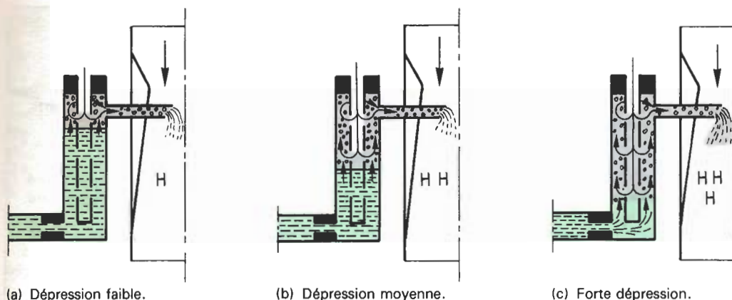
Fig. 16.14. Fonctionnement de l'émulsion étagée.
