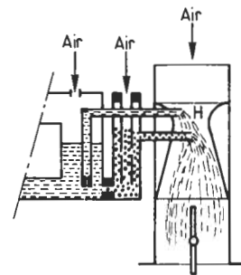
Fig. 18.3. Enrichisseur de puissance : l'économostat.
