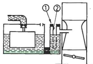
Fig. 16.12. Principe du carburateur à gicleur noyé avec mise en dérivation par tube d'émulsion étagée : 1. Ajutage d'automatisme. 2. Tube d'émulsion.
