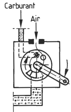
Fig. 19.7. Pivotement de la glace : position intermédiaire de ralenti accéléré.
