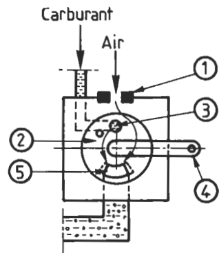
Fig. 19.6. Dispositif de starter.
