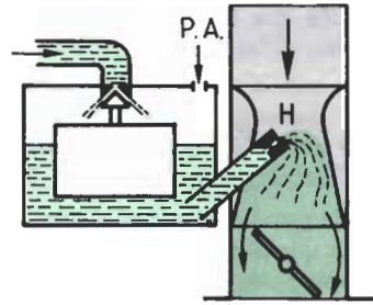
Fig. 16.6. Carburateur élémentaire.
